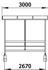
Topaz 205 - 3M
