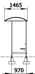
cof. słupek
