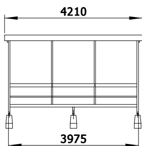
Wiata Inox Nowa 207 - 4M
