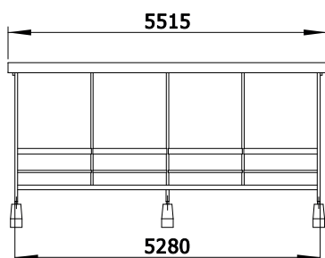
Wiata Inox Nowa 207 - 4M
