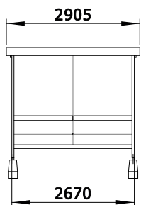
Wiata Inox Nowa 205 - 3M
